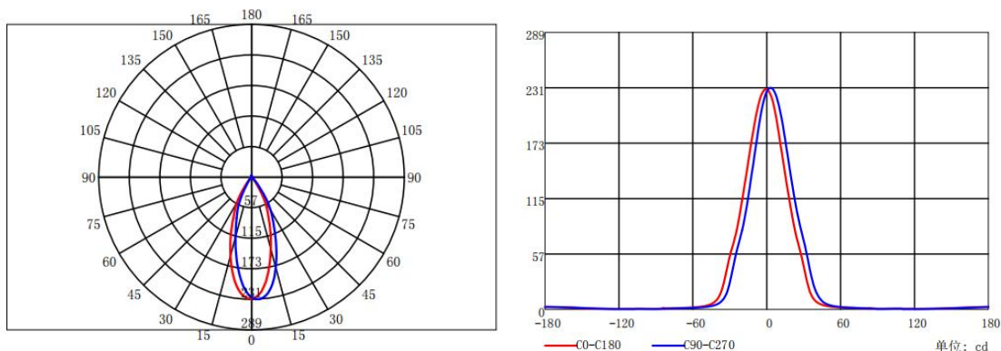
配光曲线
