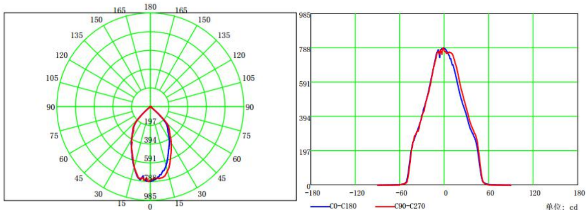
配光曲线
