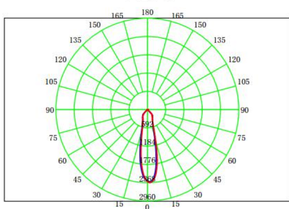
配光曲线
