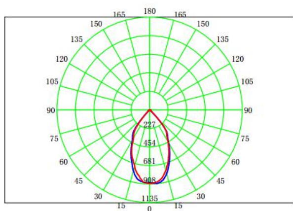
配光曲线
