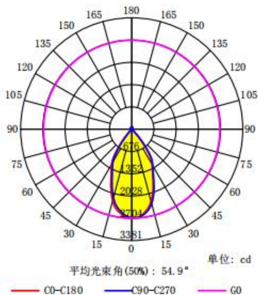
配光曲线
