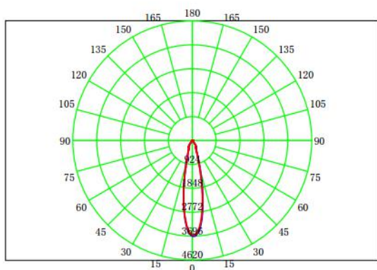
配光曲线
