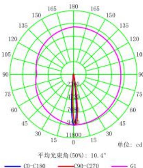
配光曲线
