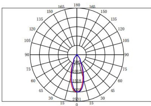
配光曲线
