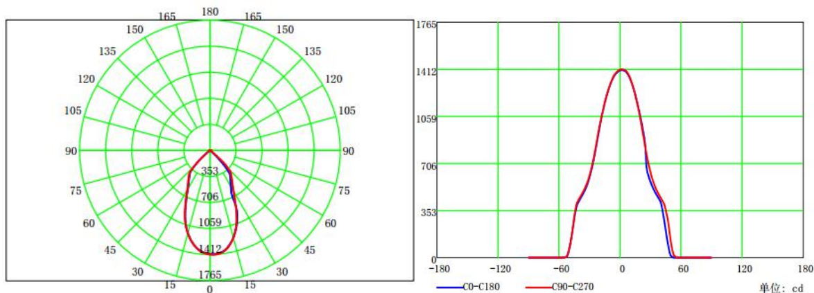
配光曲线
