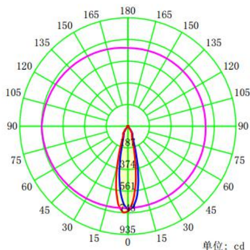
配光曲线
