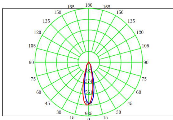
配光曲线
