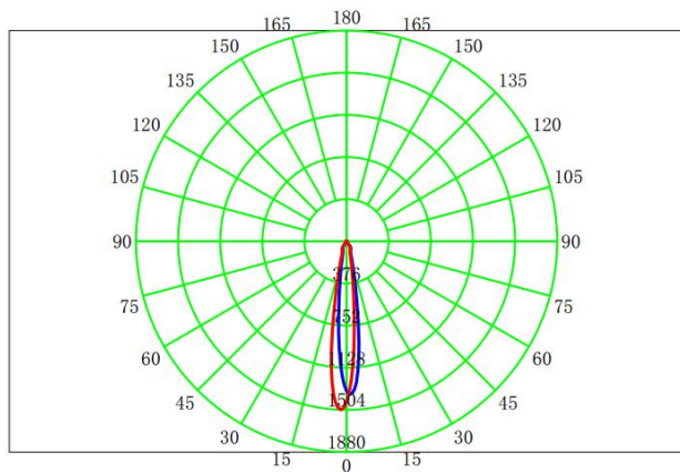
配光曲线
