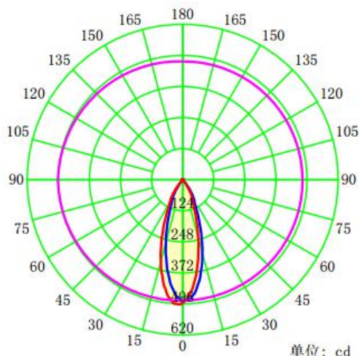
配光曲线
