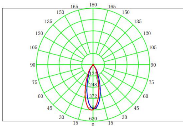
配光曲线
