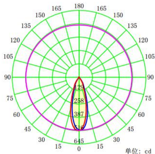
配光曲线
