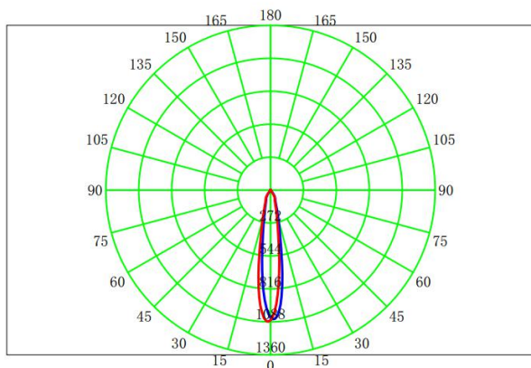
配光曲线
