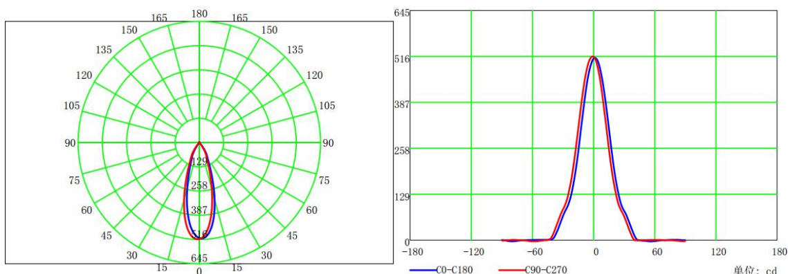
配光曲线
