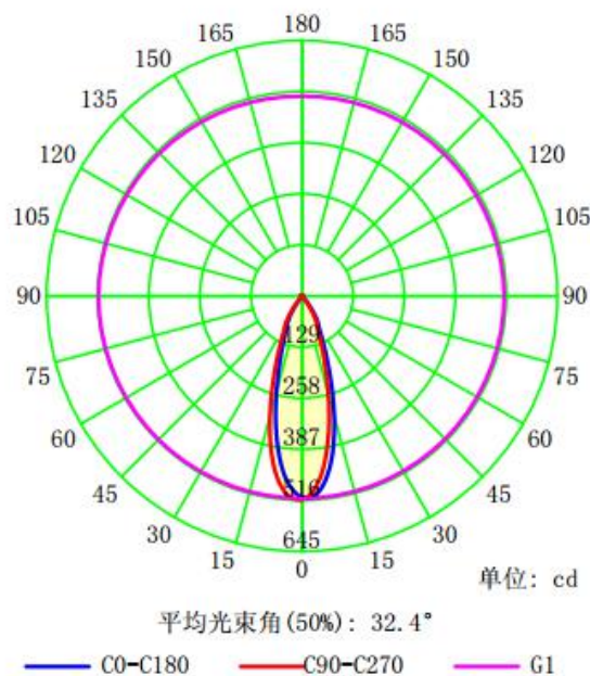
配光曲线
