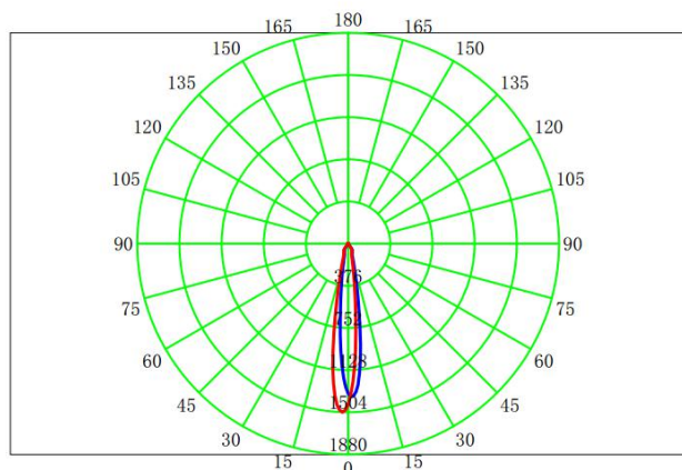
配光曲线
