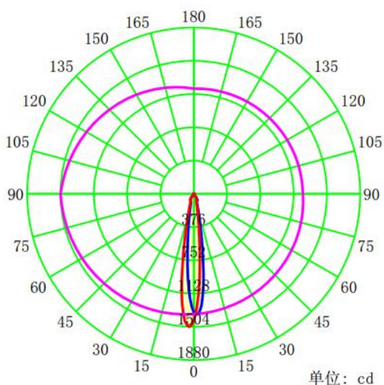
配光曲线
